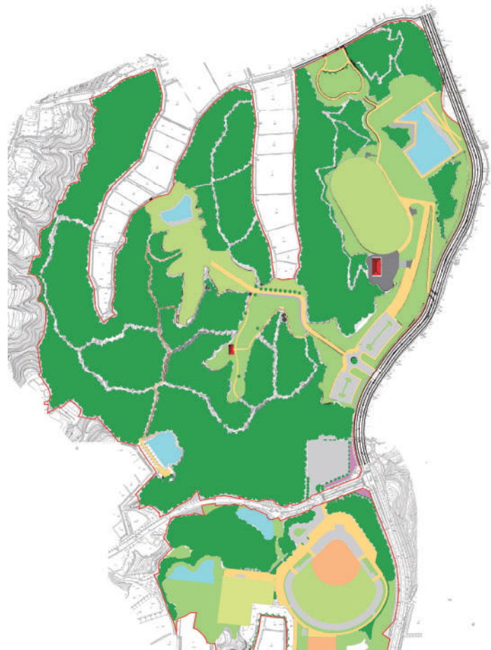
長生の森公園 施設平面図
