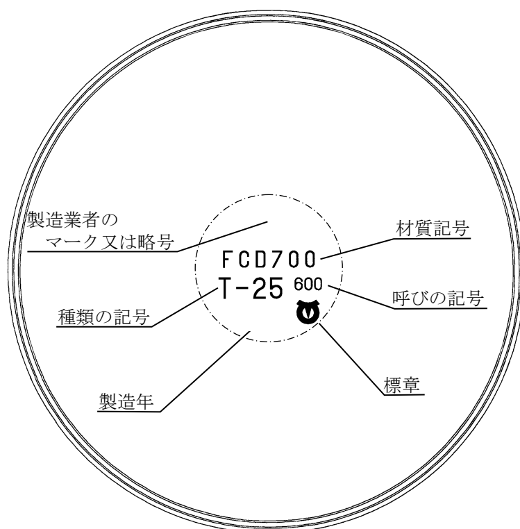
蓋裏面図
