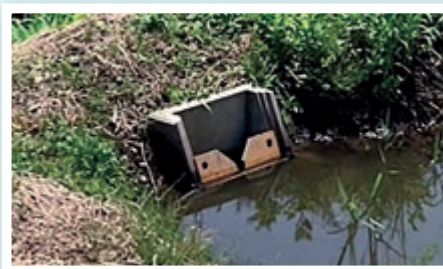
▲田んぼダムの落水桟
