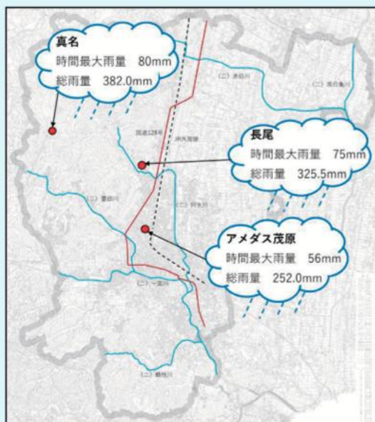
令和8年8月千葉豪雨による雨量
